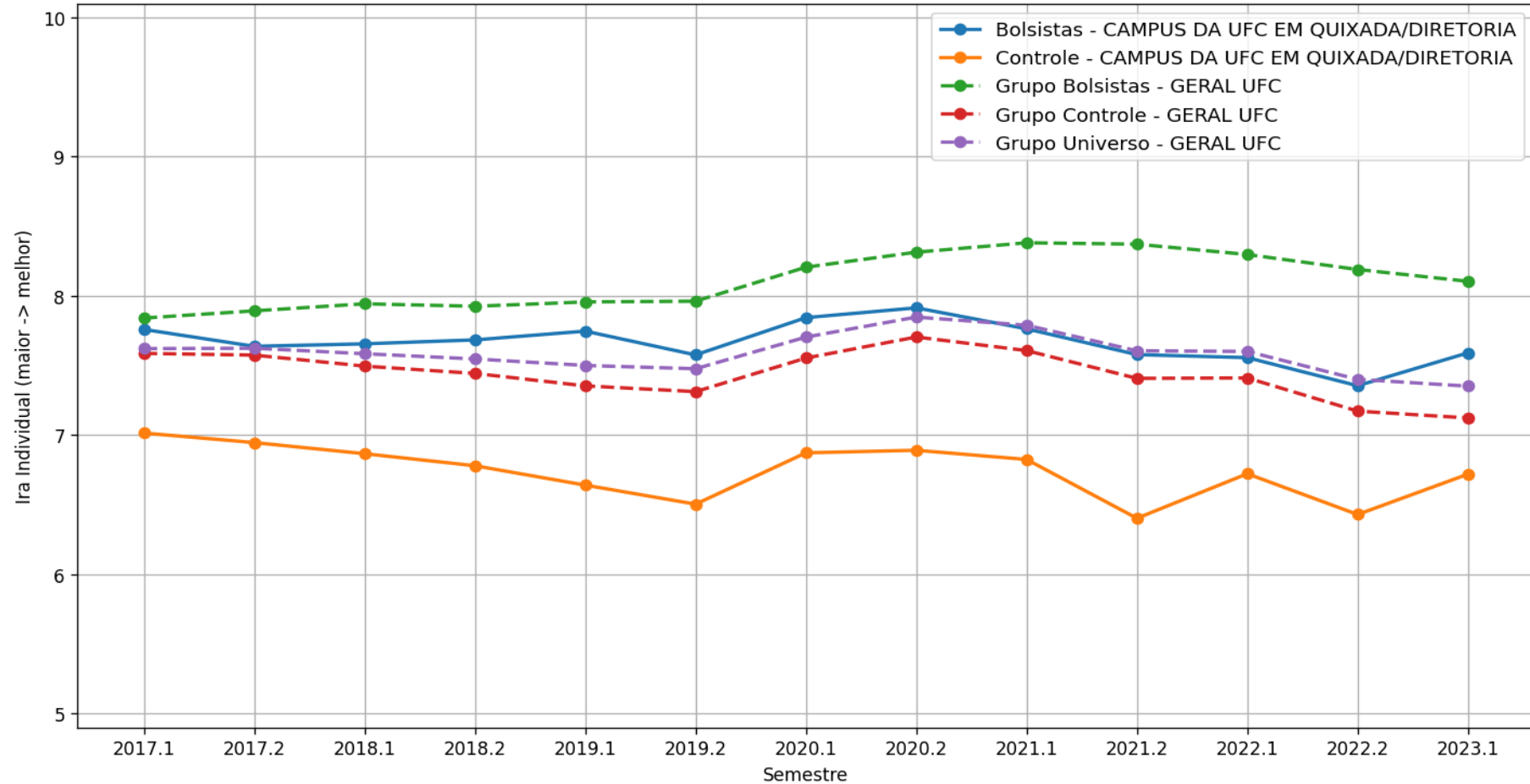
Evolução temporal do Ira Individual médio por semestre - Unid. Acadêmica - CAMPUS DA UFC EM QUIXADA/DIRETORIA
