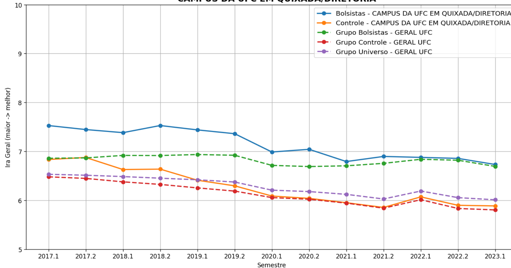
Evolução temporal do Ira Geral médio por semestre - CAMPUS DA UFC EM QUIXADA/DIRETORIA
