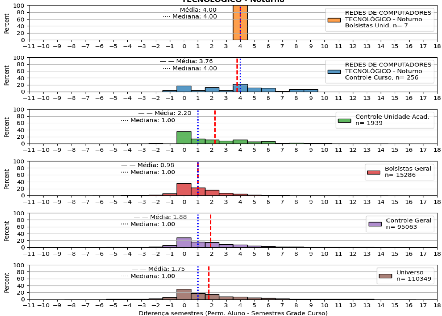
Histograma normalizado do tempo de conclusão dos alunos - Cursos - CAMPUS DA UFC EM QUIXADA/DIRETORIA REDES DE COMPUTADORES - Código Curso: 657516 TECNOLÓGICO - Noturno
